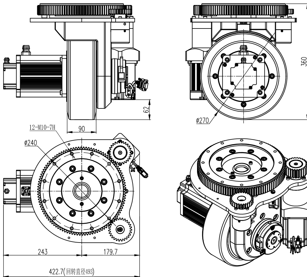
卧式舵轮ZLW-360-23008-7508-i 参数表
