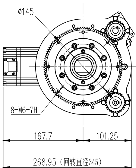
卧式舵轮ZLW-190-7508-2008-i 参数表
