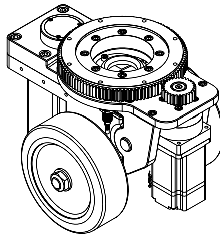
差分式舵轮ZLCW-220-7508-2008-i 参数表
